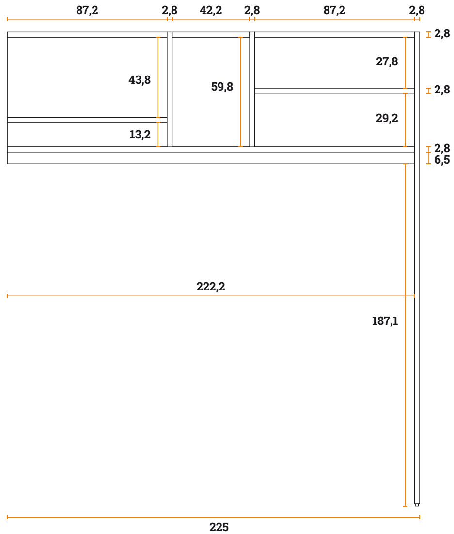
VISTA FRONTALE
