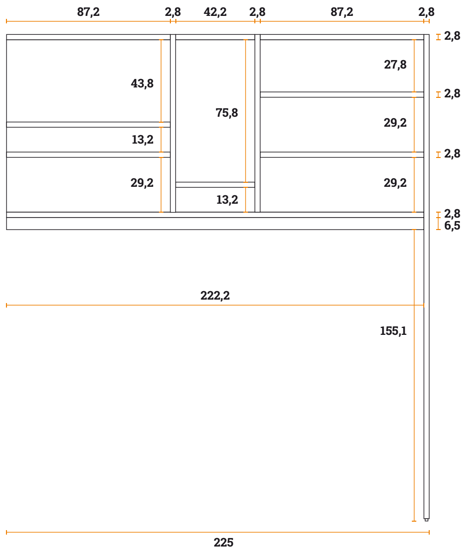
VISTA FRONTALE
