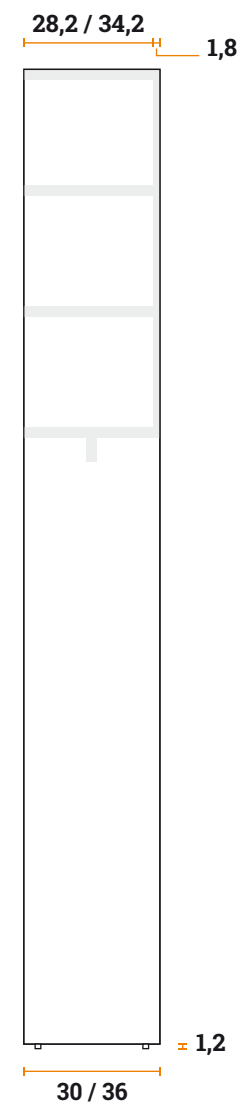
VISTA LATERALE
