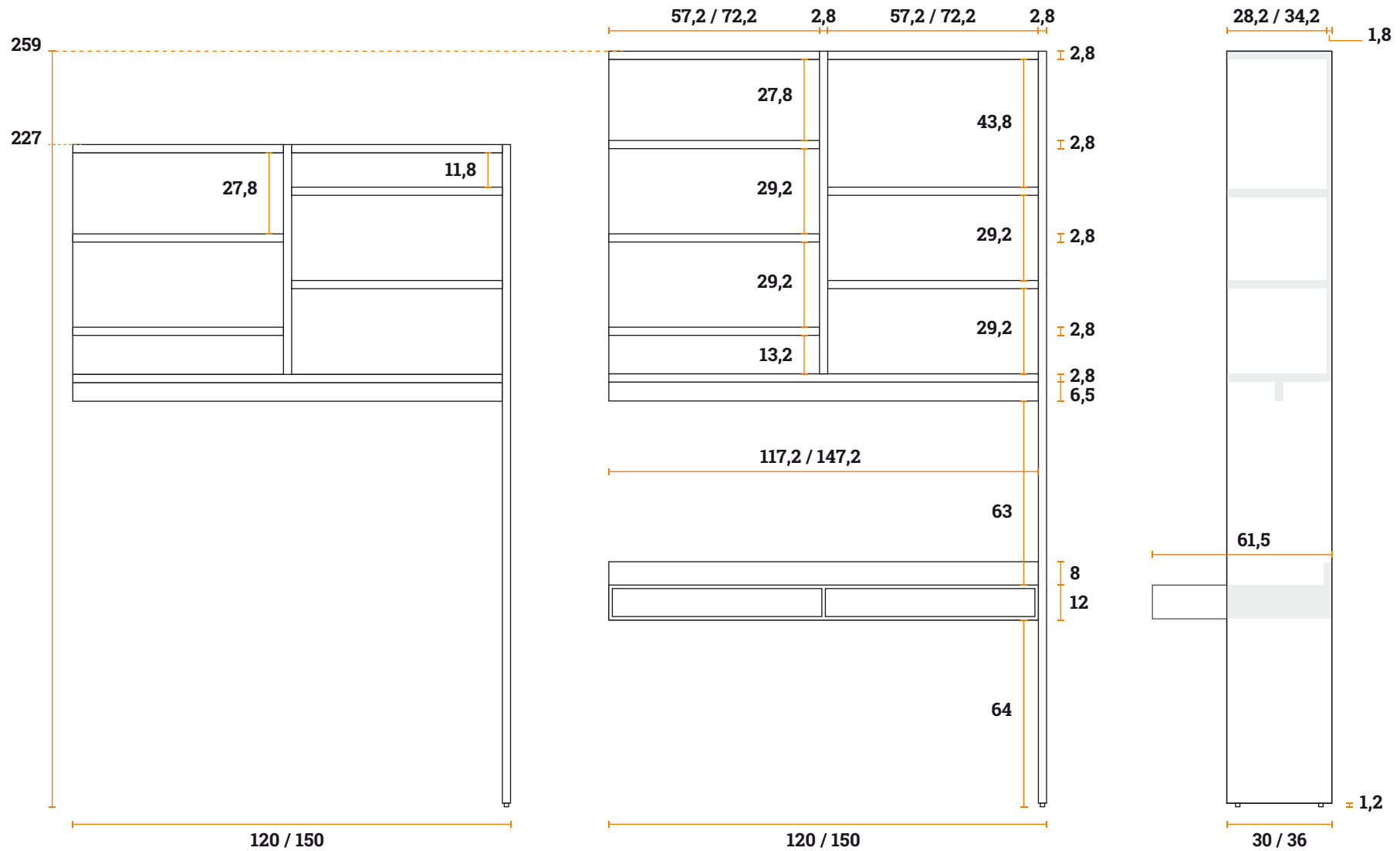
VISTA FRONTALE
