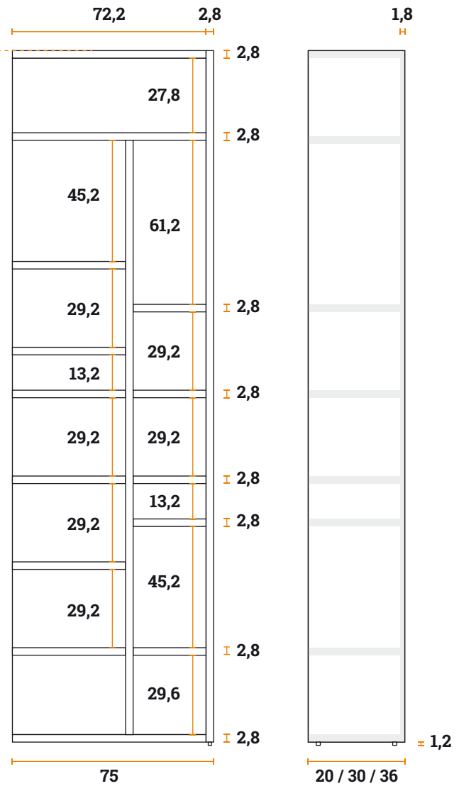
VISTA FRONTALE
