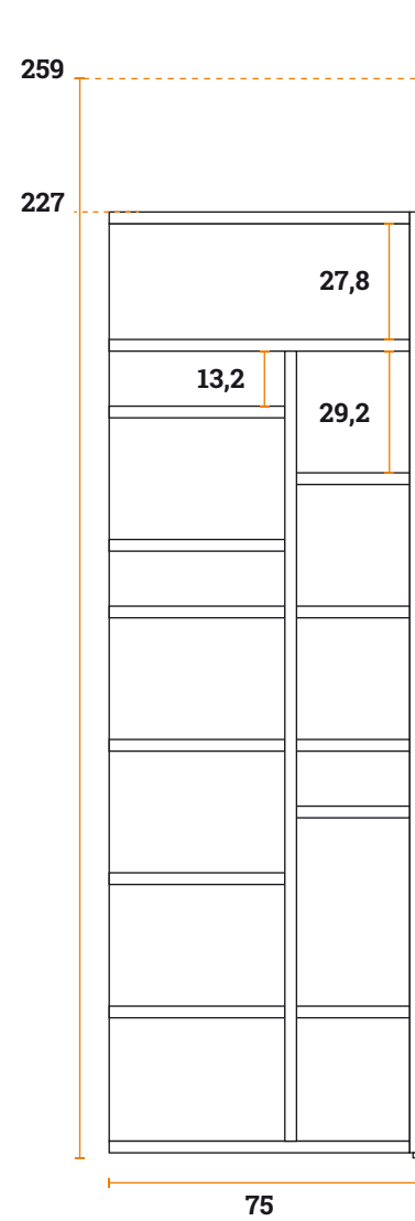
VISTA FRONTALE
