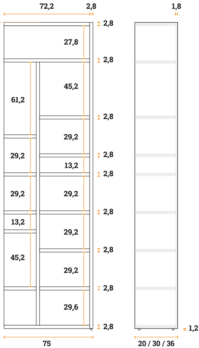
VISTA FRONTALE
